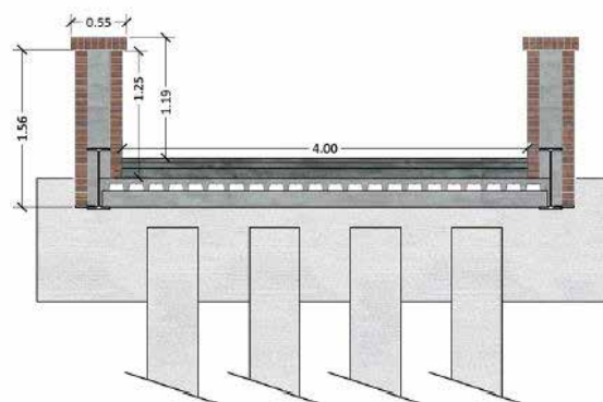
OPERE DI CONSOLIDAMENTO DI UN PONTE SU CORSO D'ACQUA LUNGO IL TRACCIATO STRADALE SEZIONE - SCALA 1:20
